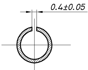
CORTE C-C
